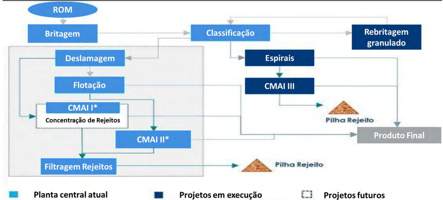
Figura 3: Fluxograma atual para a Planta Central e projetos em desenvolvimento
