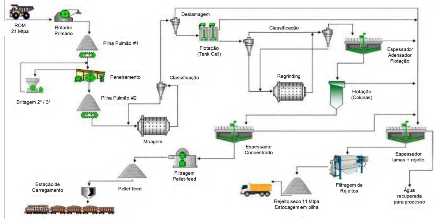
Figura 9: Fluxograma da P15 Itabirito
